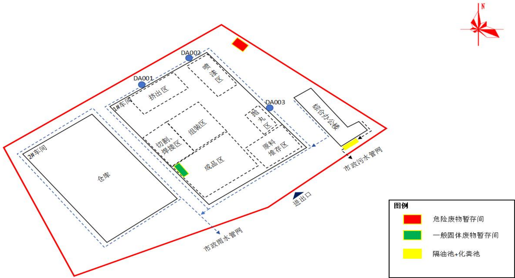
附图3 项目总平面布置图及雨污管网图
