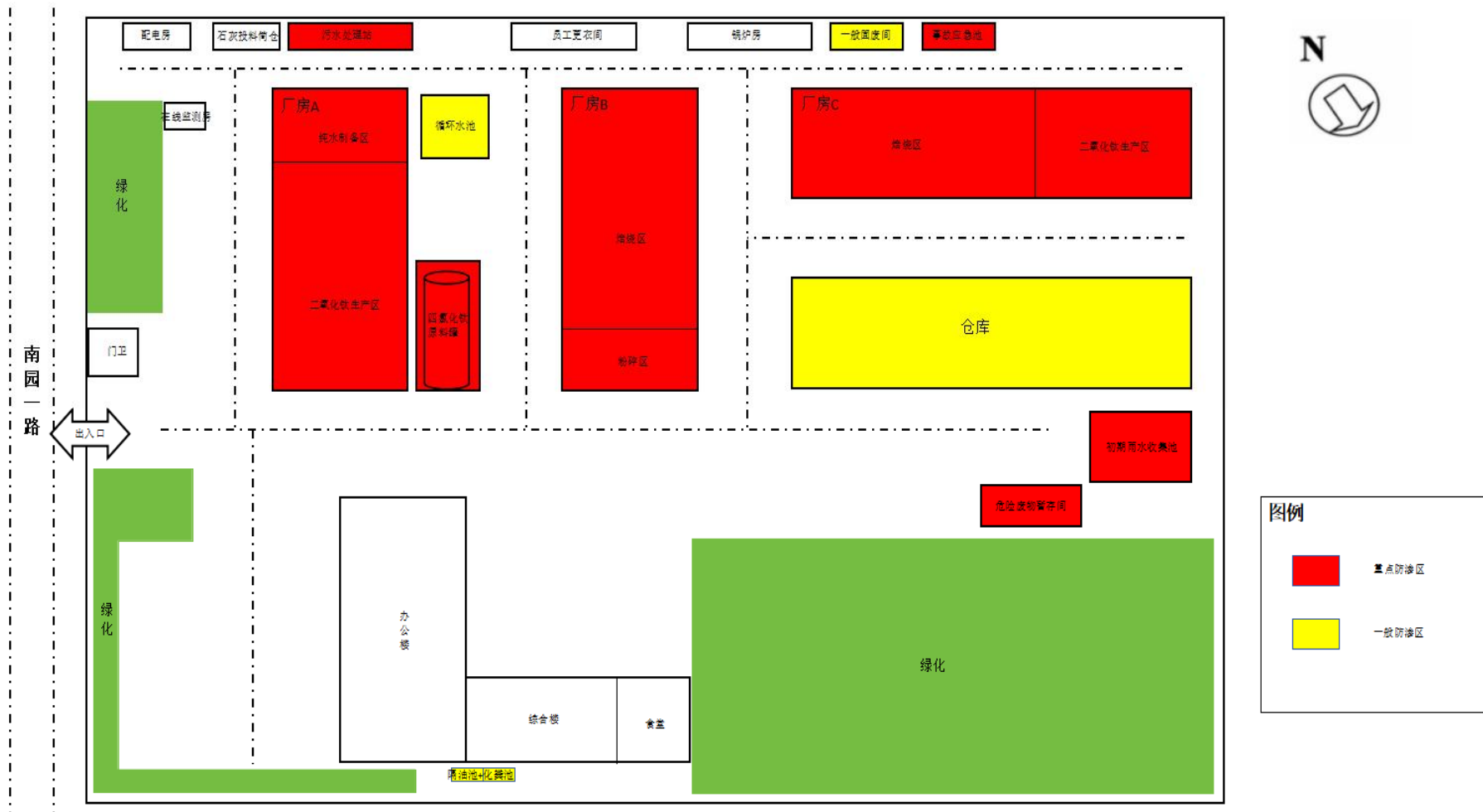
附图6 项目分区防渗图
