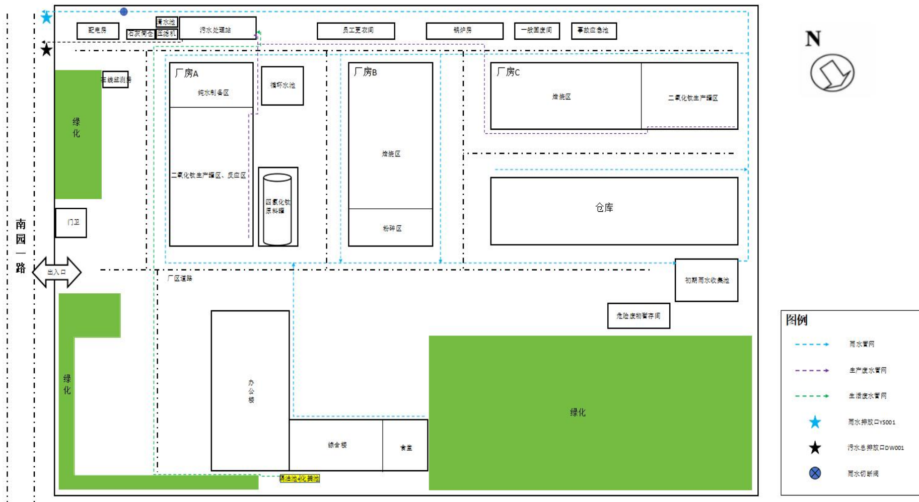
附图 5 项目厂区雨污管网图
