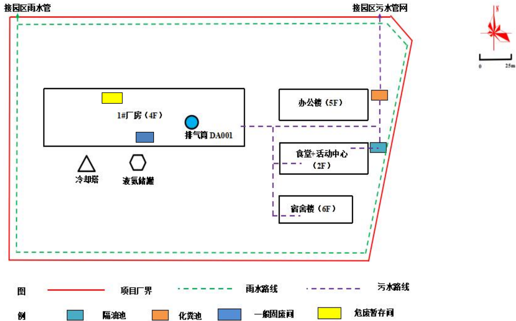
附图 3-1 项目总平面布置及雨污管网图
